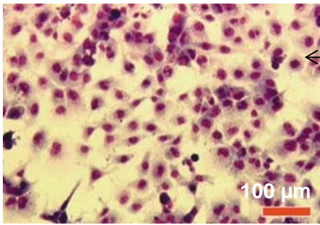
Photographie A : l’expression du gène de la syncytine est inactivée.
