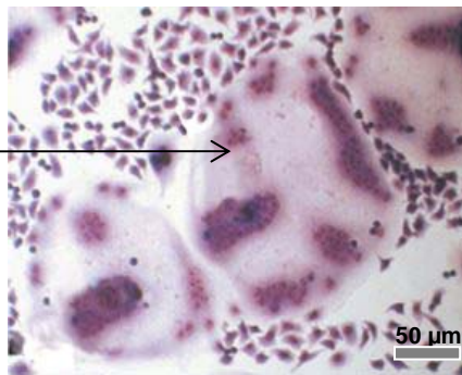
Photographie D : l’ADN des cellules a intégré la séquence ENV du virus.
