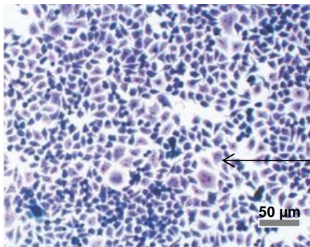
Photographie C : l’ADN des cellules ne contient pas la séquence ENV du virus.
