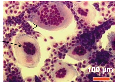
Photographie B : l’expression du gène de la syncytine est activée.
